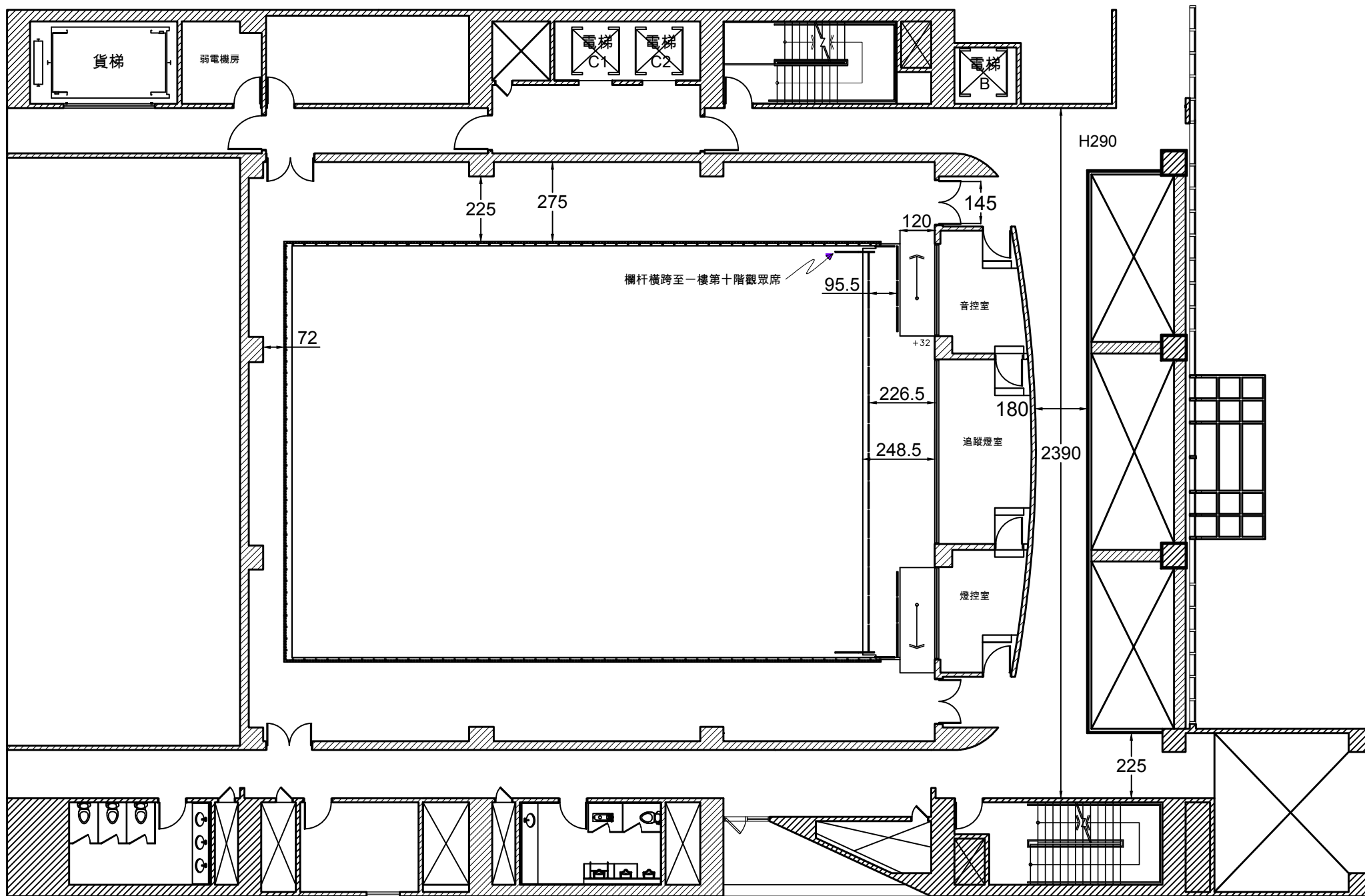
圖 (四) 小表演廳_2F空間平面圖 (單位：公分) Figure(4) Experimental Theatre_2 nd Floor Plan (Unit: cm)
